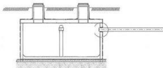
Szamba betonowe dwukomorowe
